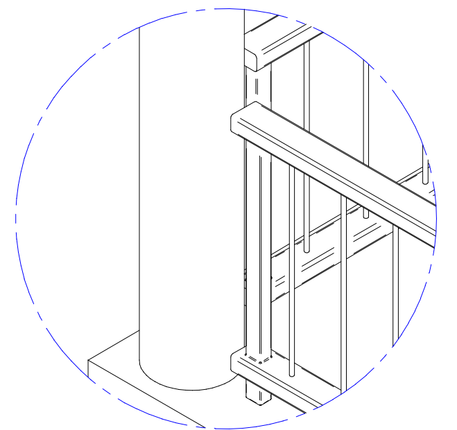
DETAIL A 2:1
